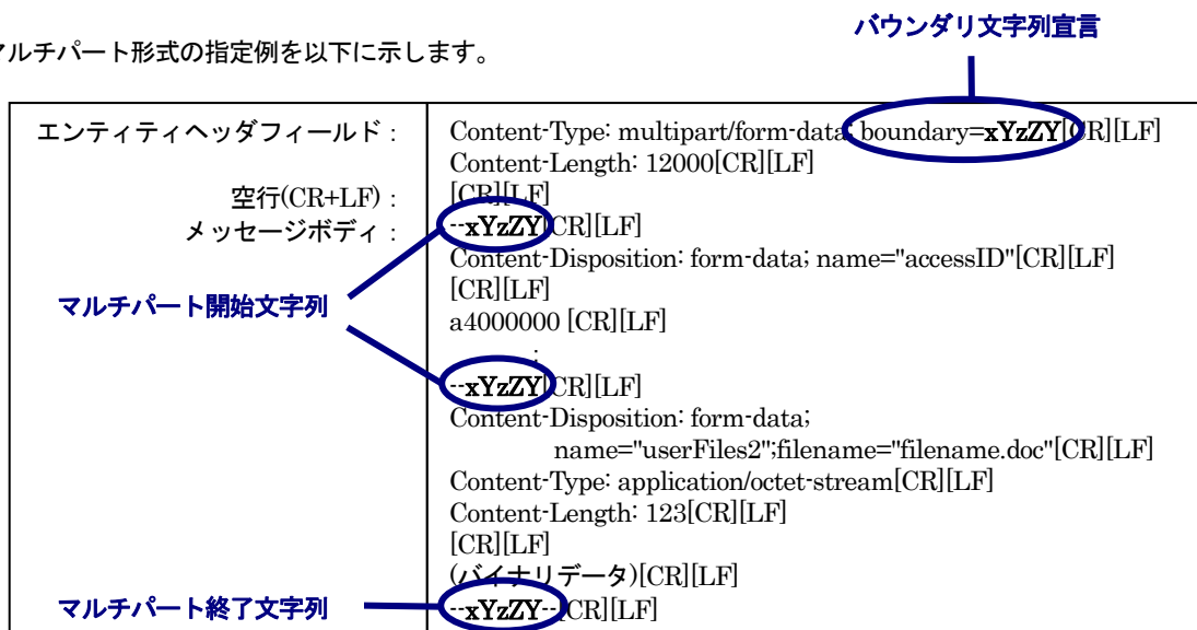
図 3-1 マルチパート形式の指定例
