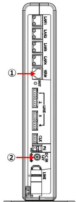
本装置 SG2000is4/is8 背面図
