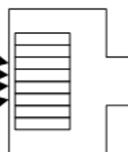
LANケーブル/RJ-45コネクタ側の配線 (RJ-45コネクタを先端から見た図)
